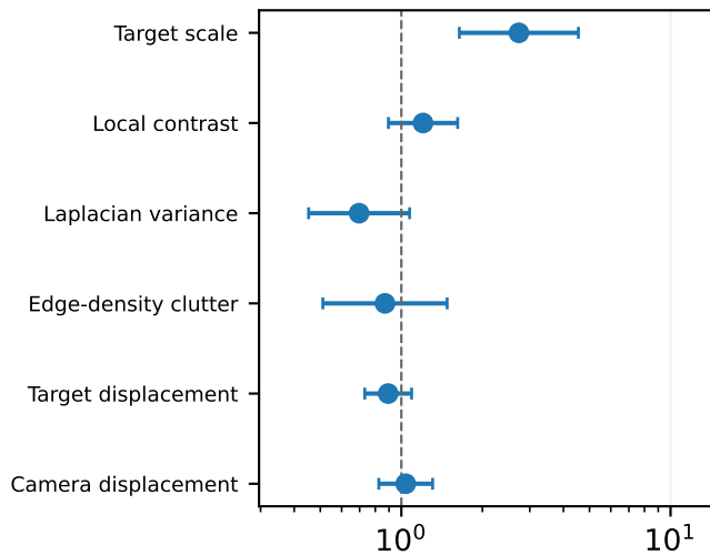
YOLOv8s
