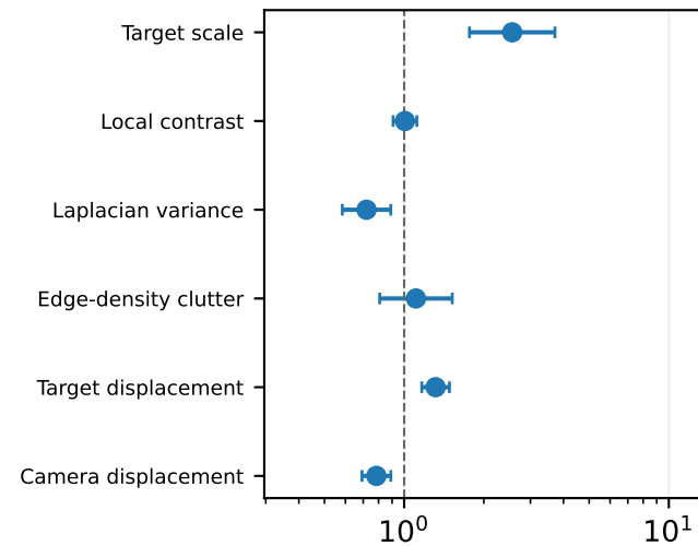
YOLOMG-Arch
