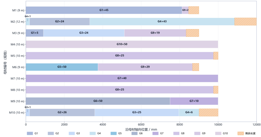
图 6: 问题二共切优化结果示意图
