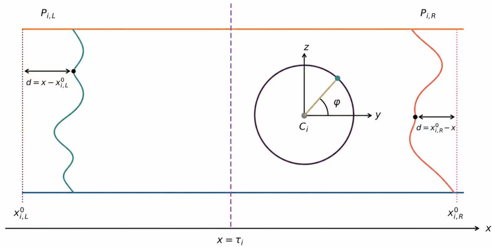
图 4: 端部点云划分与缩进距离构造示意图
