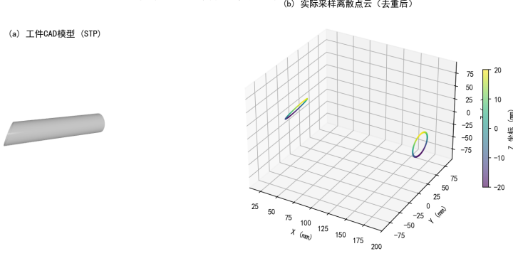
图 2: 圆管 1 点云与 STP 文件对比图
