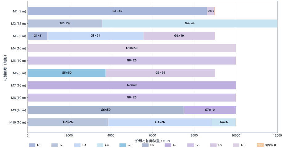
图 3: 问题一优化结果示意图
