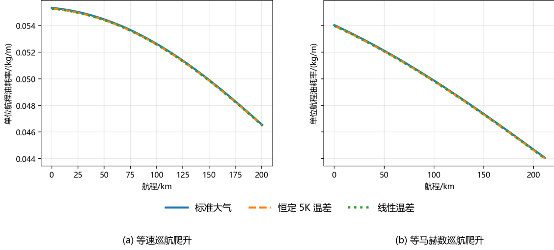
图 5: 温度偏差修正前后单位航程油耗率对比
