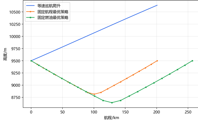
图 7: 等速策略与最优策略高度剖面对比
