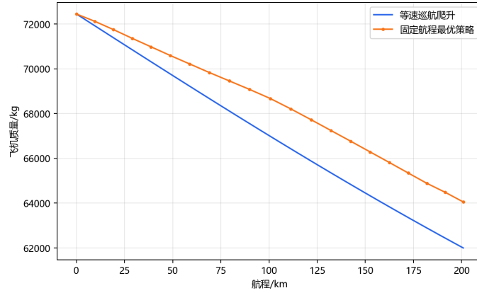
图 9: 固定航程条件下等速策略与最优策略节油效果对比
