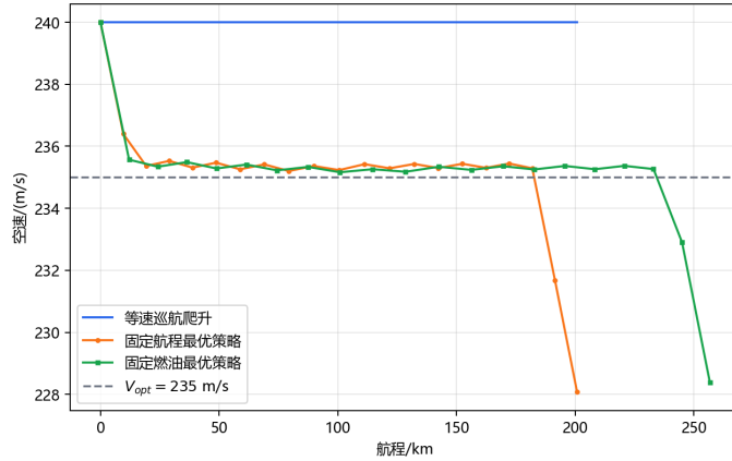
图 8: 固定航程最优策略的高度、速度、质量与油耗率演化对比
