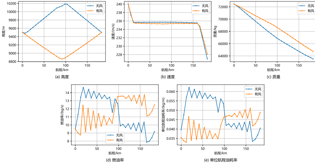
图 6: 无风与有风条件下高度、速度、质量、燃油率和单位航程油耗率对比图
