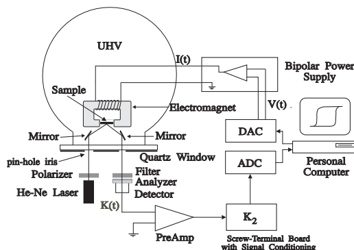
电路图
