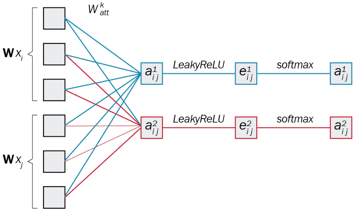
교재 그림 7.2: 여러 attention head의 결과를 결합하는 흐름
