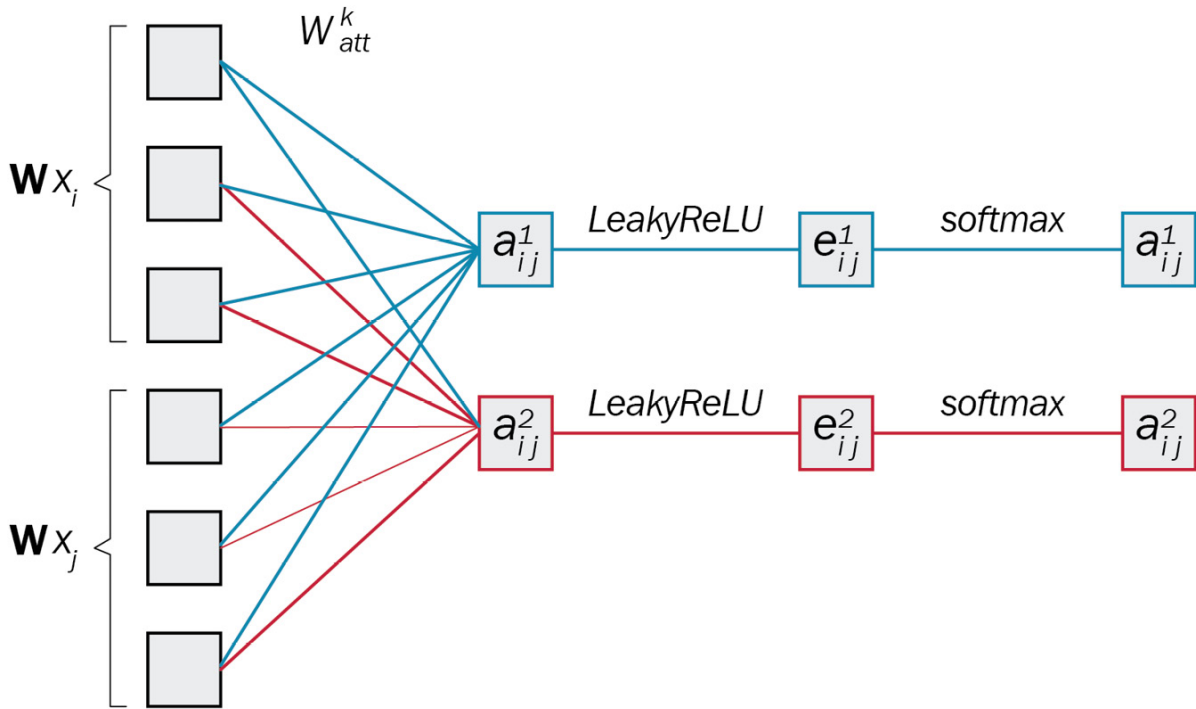
Figure 7.2 (교재): 계수 정규화와 메시지 집계
