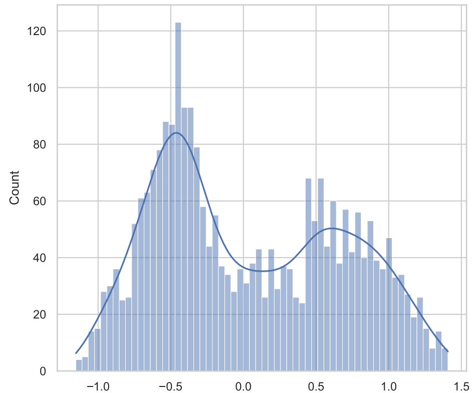
u error
