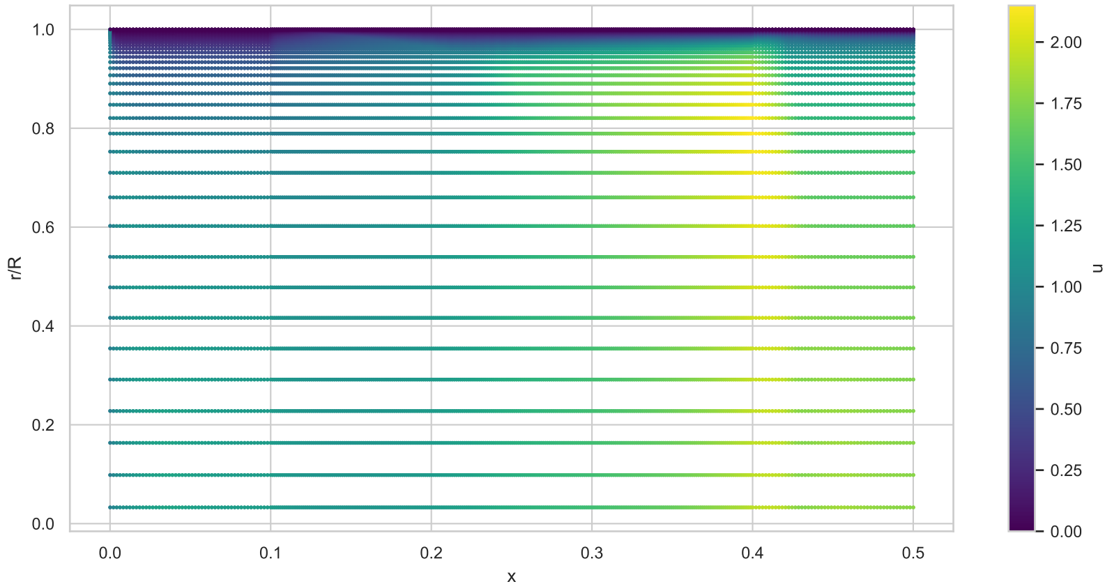
u cloud (1.5-473-500)
