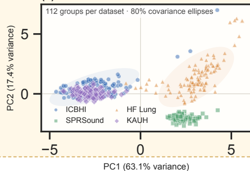
(b) Acoustic-feature PCA
