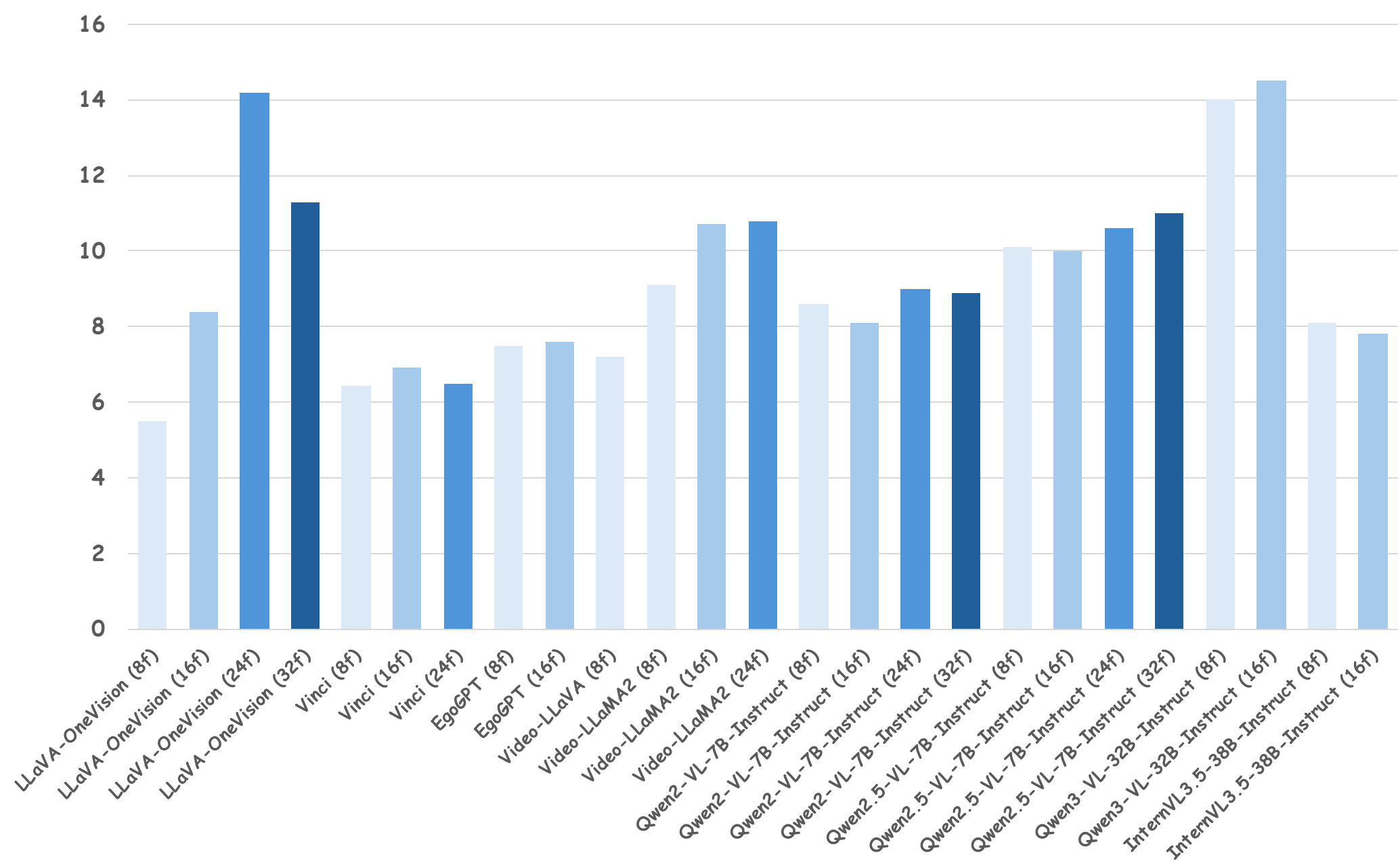
(b) Precision
