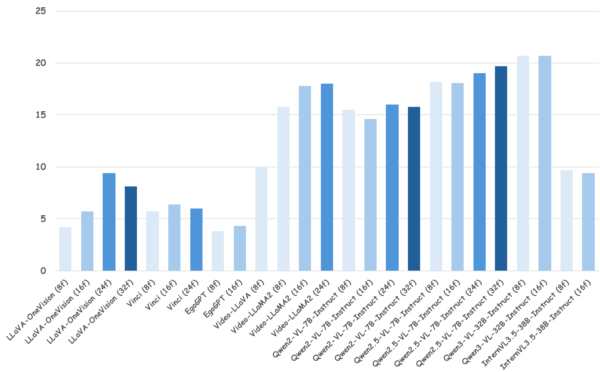
(d) F1
