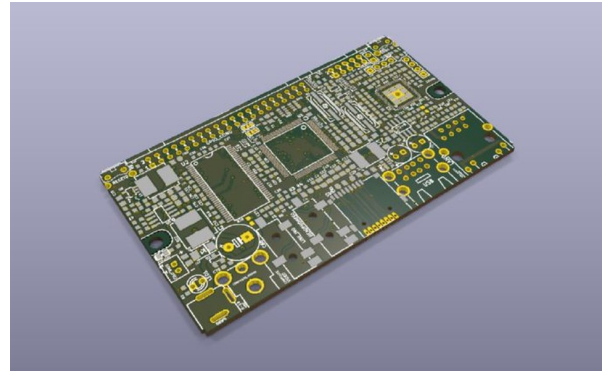
iMX233-OLinuXino-MAXI Rev D (Olimex)
