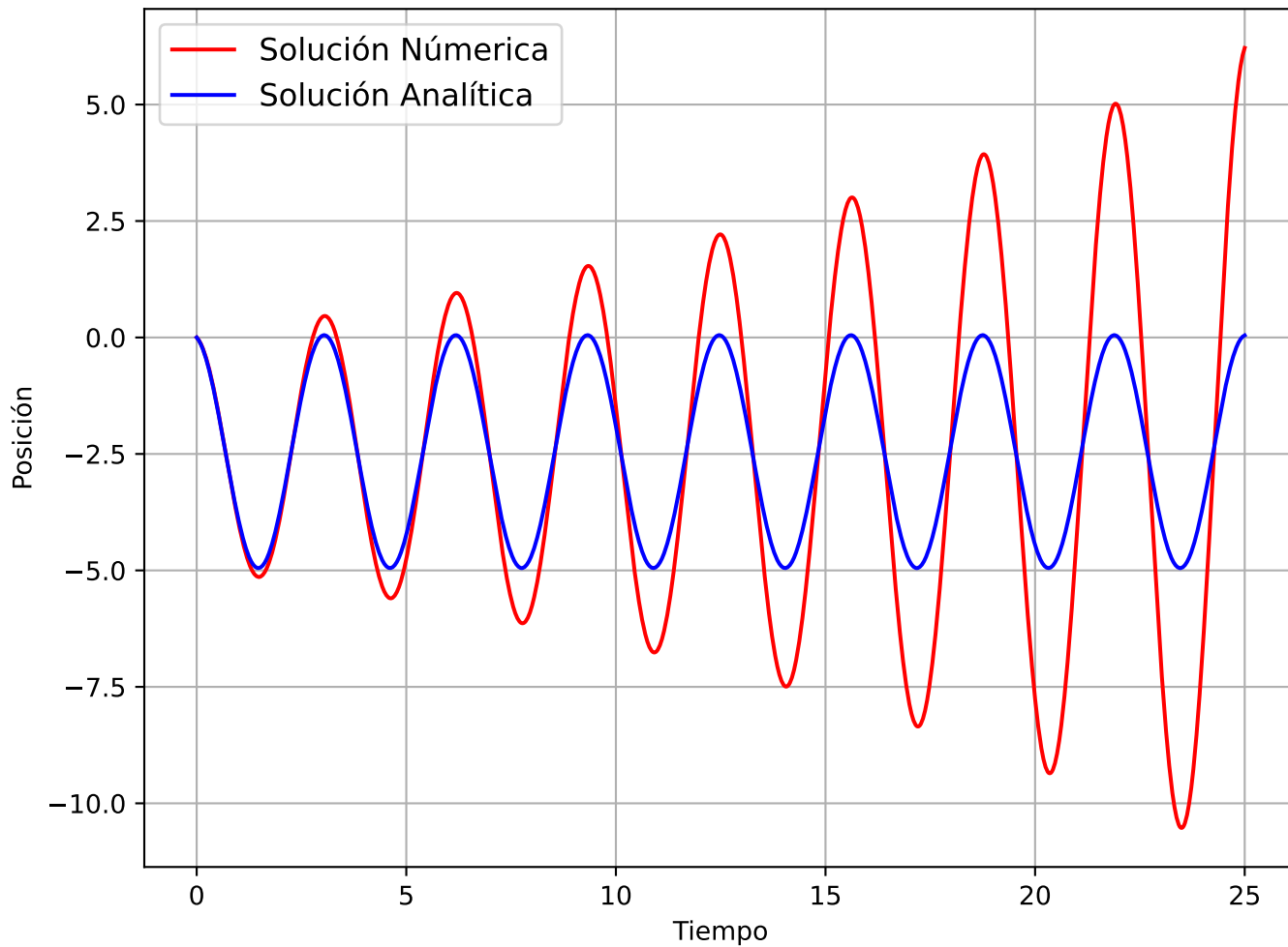
Solución Numérica vía Método Euler
