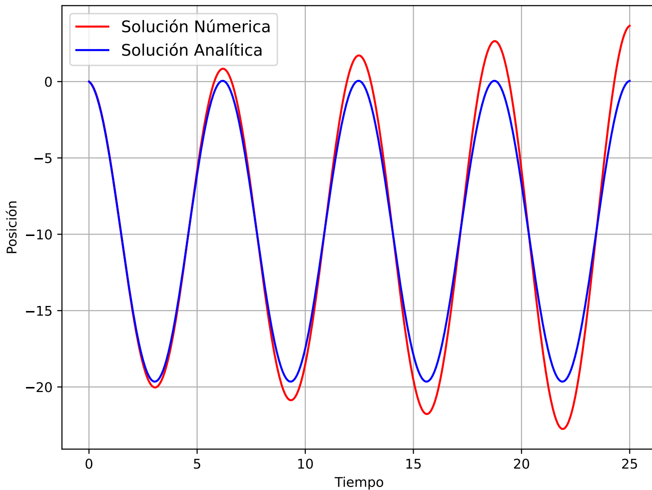
Solución Numérica vía Método Euler
