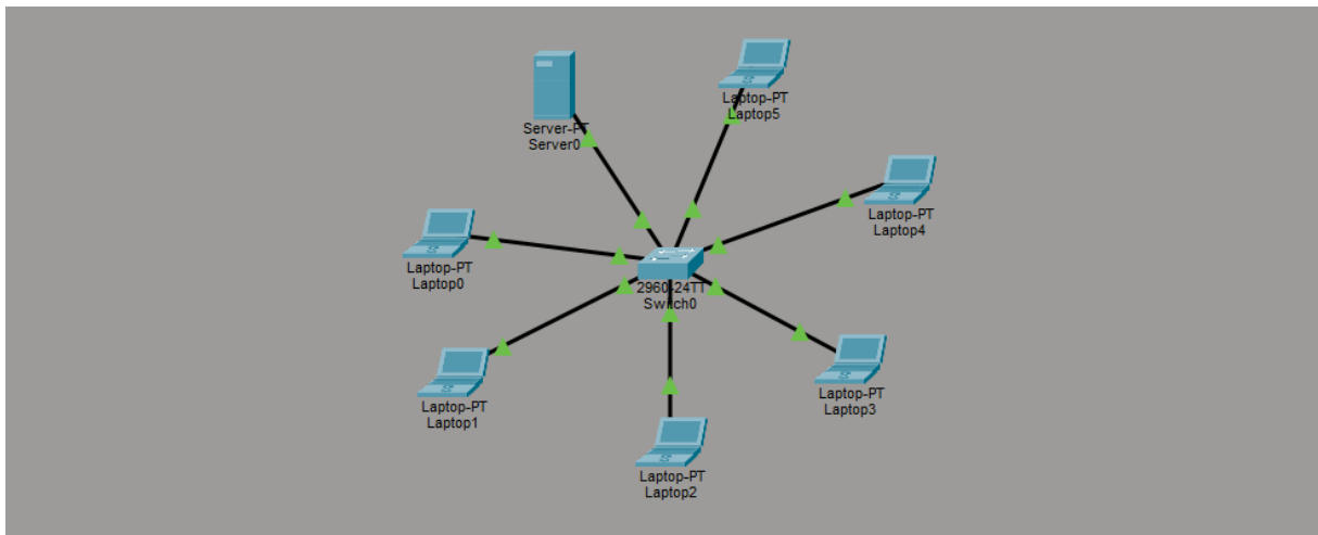
FIGURA 2 – Topologia lógica do sistema de monitoramento.
