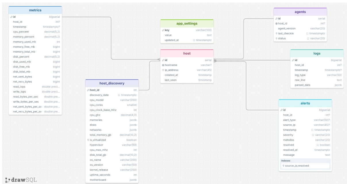
FIGURA 11 – Modelo lógico do banco de dados.
