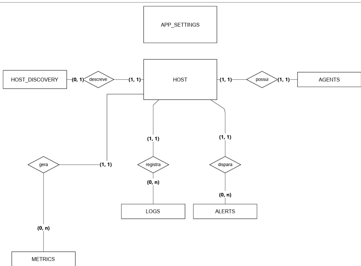
FIGURA 10 – Modelo conceitual (entidade-relacionamento) do banco de dados.
