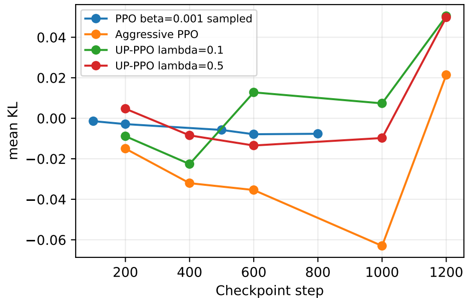
Approximate KL trajectory
