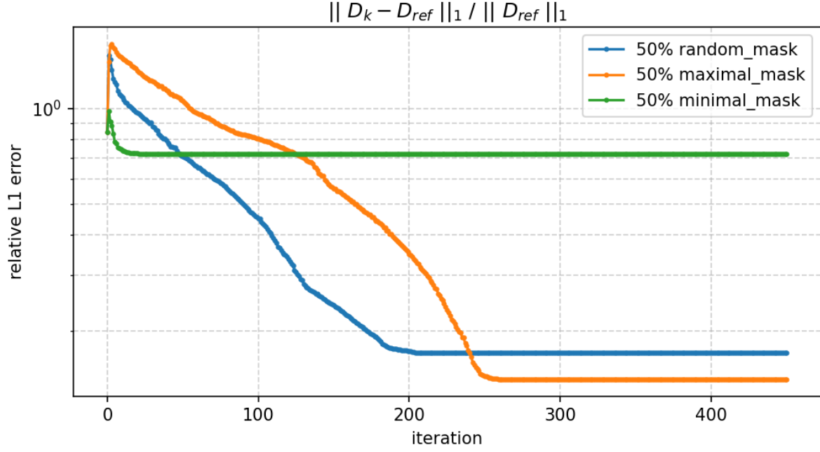
Рис. 4: Относительная ошибка восстановления матрицы (выбор наблюдаемых рёбер: top/bottom/random)
