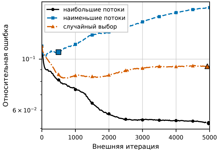
(а) Ошибка полного потока E_{full}
