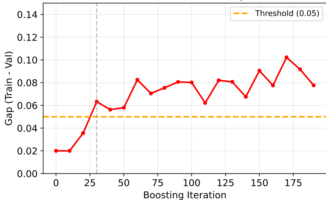
(d) Adaptive min_child_weight
