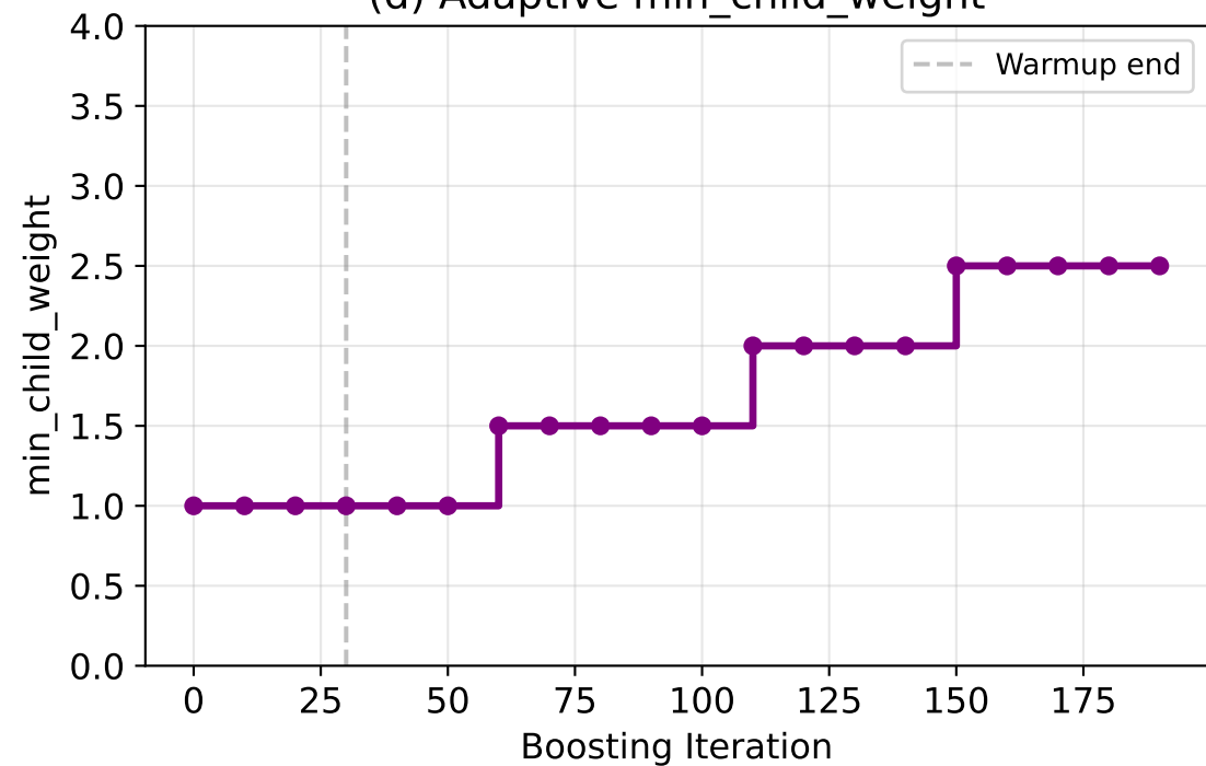
(d) Adaptive min_child_weight
