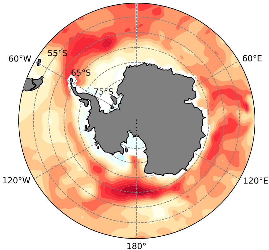
D (CESM2-NUDGE)
