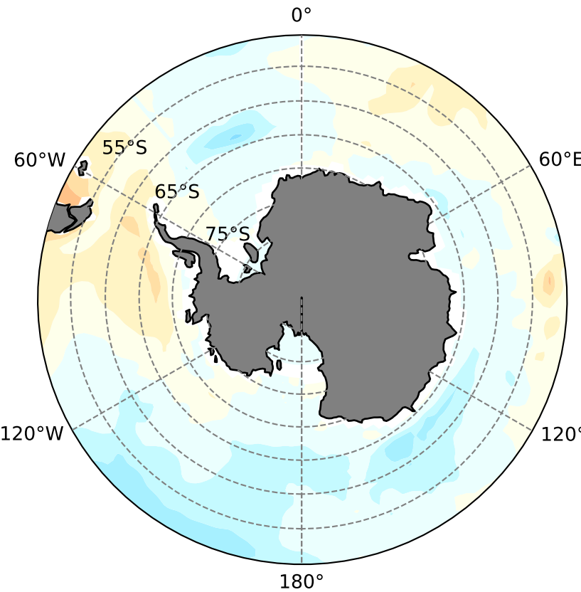
\Delta Max (1998)
