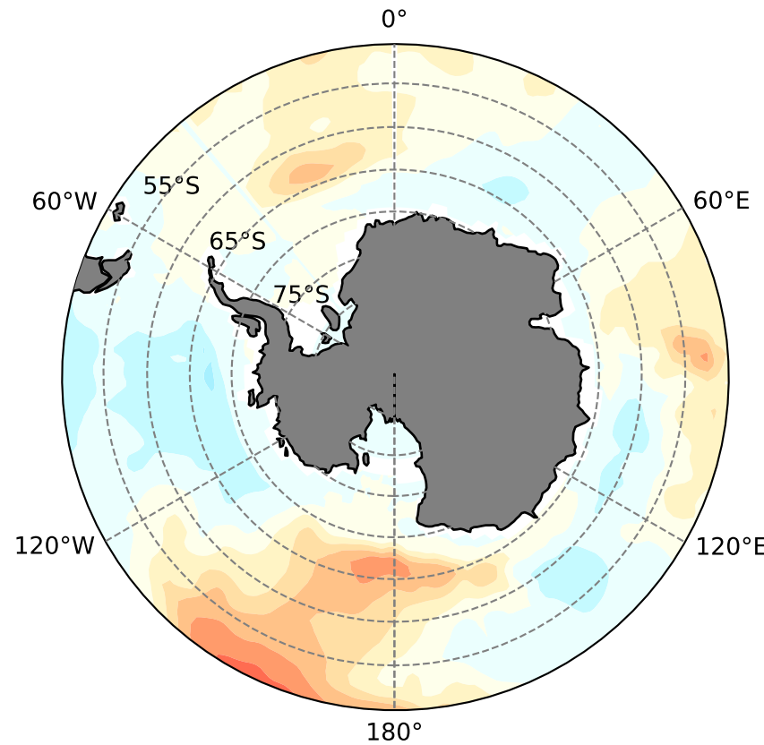
\Delta 2023
