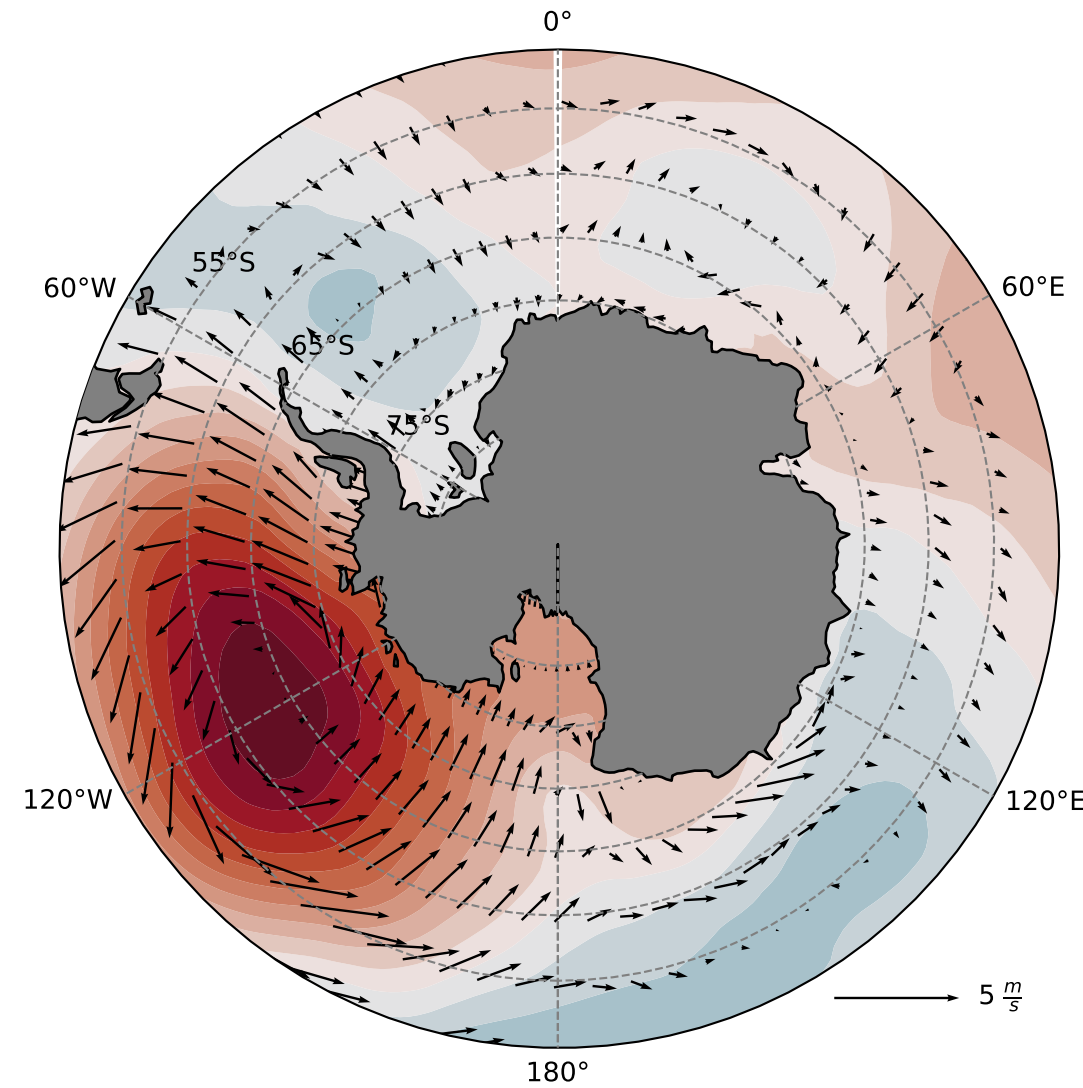
ERA5 Nino-Nina
