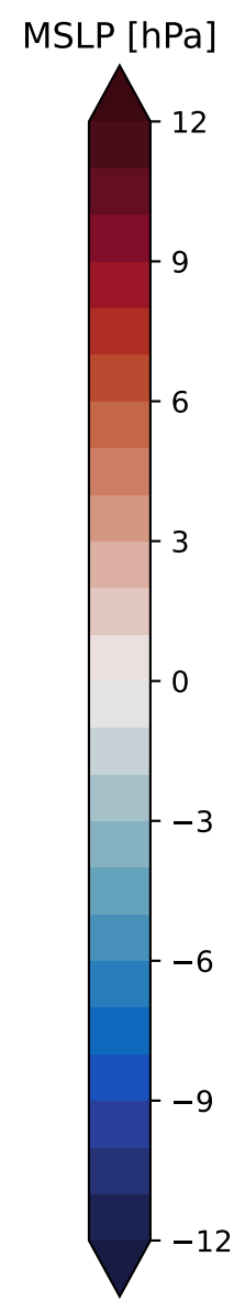
ERA5 Nino-Nina
