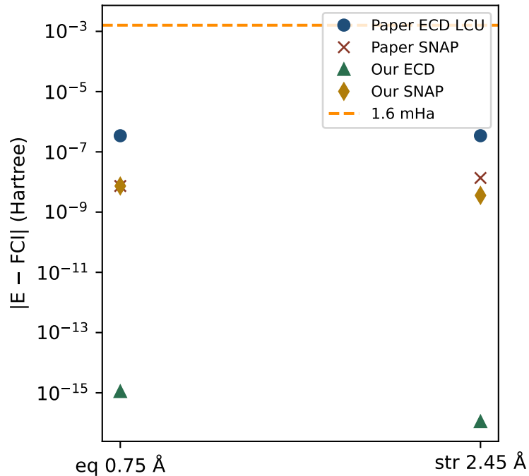
Error vs FCI
