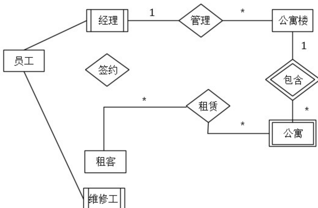
图2-1 实体联系图
