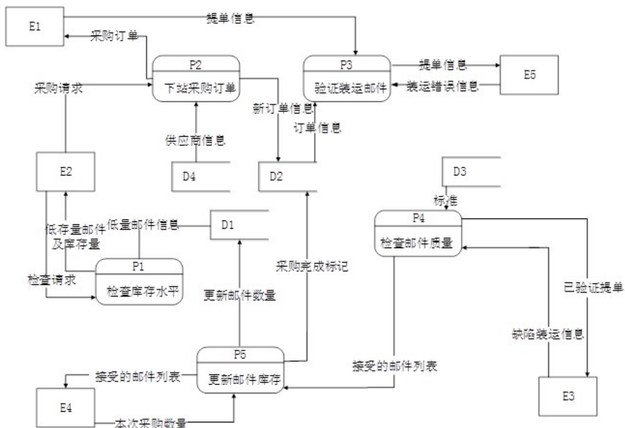
图 1-2 0层数据流图
