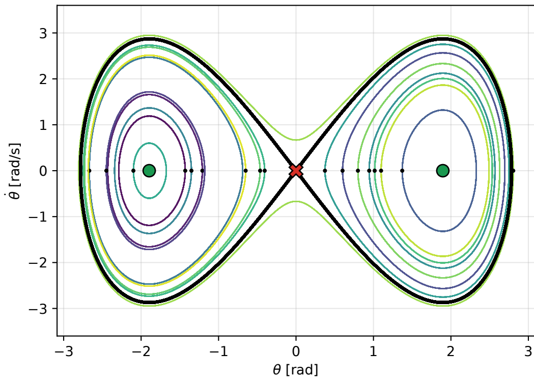
Separatrix, k = 0.5 k_{cr}
