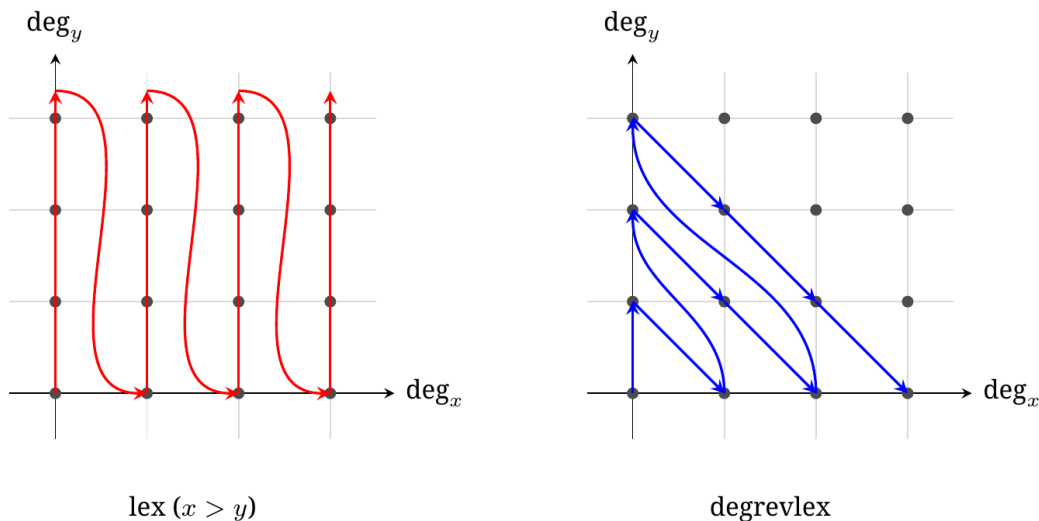
Σχήμα 5: Σύγκριση lex και degrevlex στο μονοειδές όρων [x, y] (με x > y ): τα βέλη δείχνουν τη φορά αύξησης. Η lex διατρέχει στήλη-στήλη (πρώτα ο εκθέτης του x )· η degrevlex διατρέχει διαγώνιο-διαγώνιο (πρώτα ο ολικός βαθμός).
