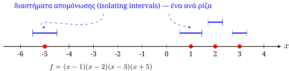
Σχήμα 3: Απομόνωση των τεσσάρων πραγματικών ριζών του f = (x - 1)(x - 2)(x - 3)(x + 5) σε ξένα μεταξύ τους διαστήματα.
