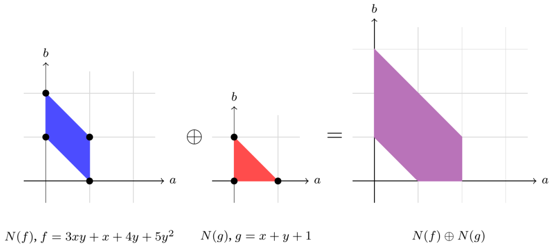
Σχήμα 4: Τα πολύτοπα Newton N(f), N(g) δύο πολυωνύμων και η άθροισή τους Minkowski N(f) \oplus N(g) — η γεωμετρική κατασκευή πάνω στην οποία στηρίζεται το θεώρημα BKK.
