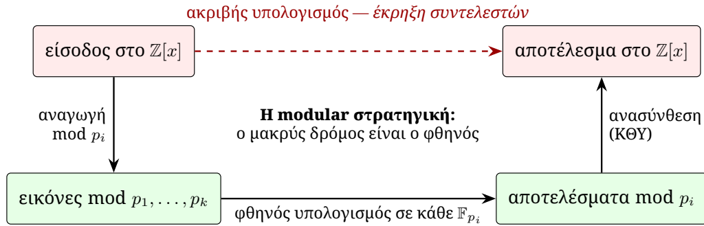
Σχήμα 3: Η modular στρατηγική. Ο άμεσος (διακεκομμένος) δρόμος πάνω από το \mathbb{Z} υποφέρει από έκρηξη των ενδιάμεσων συντελεστών· ο “μακρύς” δρόμος — αναγωγή modulo πολλούς πρώτους, φθηνός υπολογισμός σε κάθε \mathbb{F}_{p_i} , ανασύνθεση με ΚΘΥ — είναι στην πράξη ο φθηνός.
