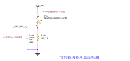
电机驱动芯片温度检测
