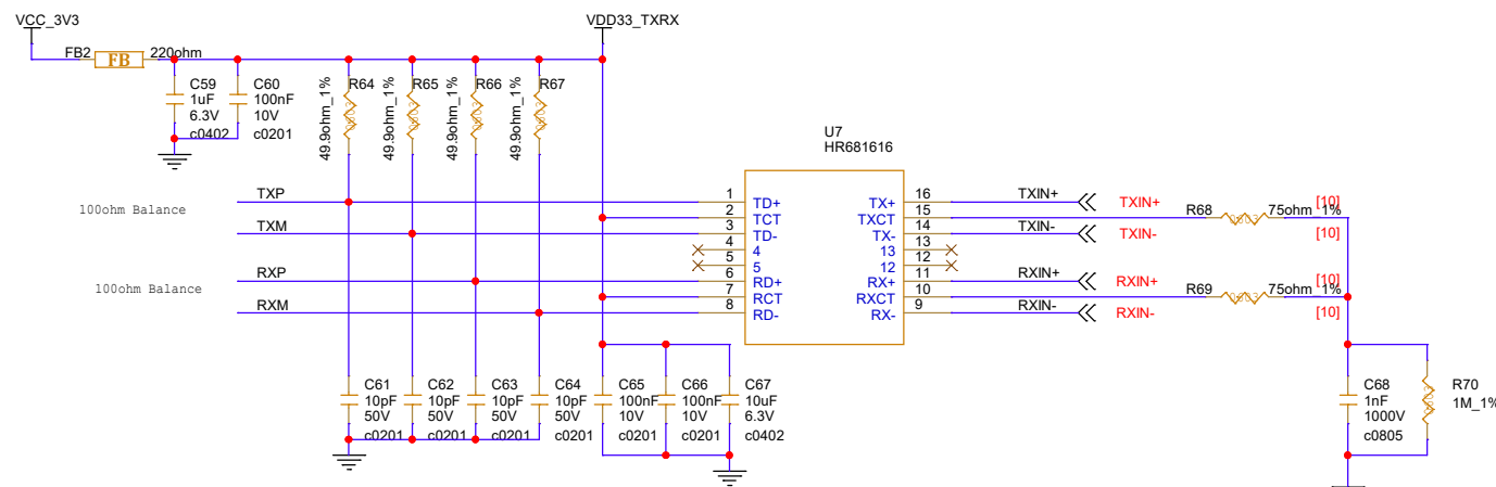
网络变压器电路
