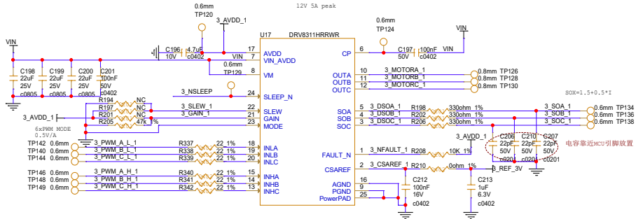
电机驱动电路
