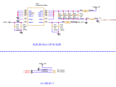
MCU烧录口
