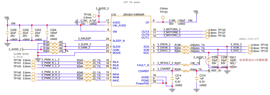
电机驱动电路
