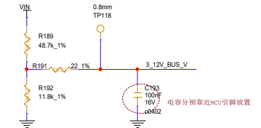
电机母线电压12V检测
