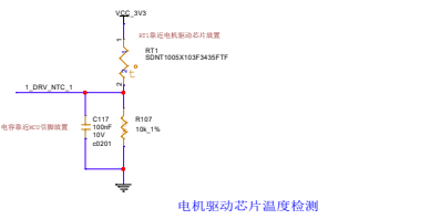
电机驱动芯片温度检测
