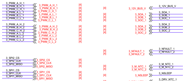
与8T2连接网络
