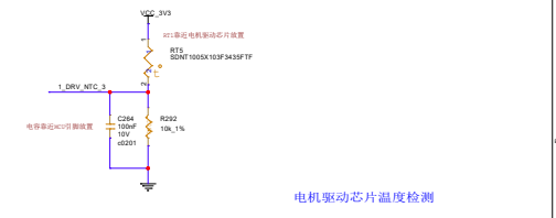
电机驱动芯片温度检测
