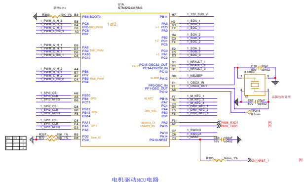
电机驱动MCU电路
