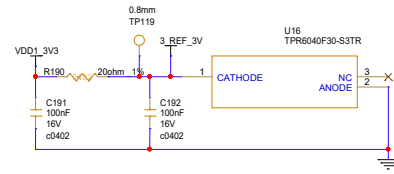
ADC基准电压
