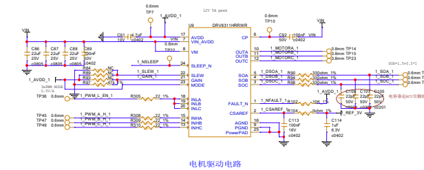
电机驱动电路
