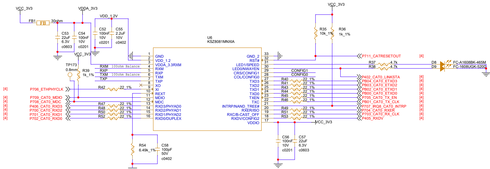
PHY电路
