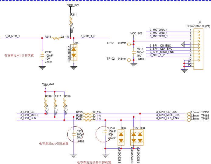
电机及编码器接口
