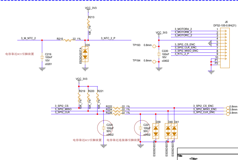
电机及编码器接口
