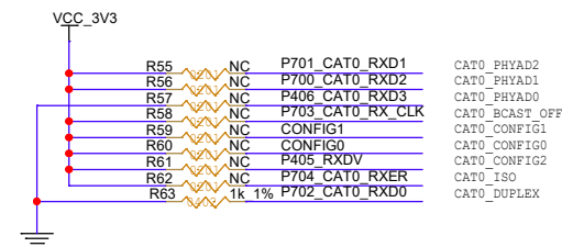
PHY配置预留电路
