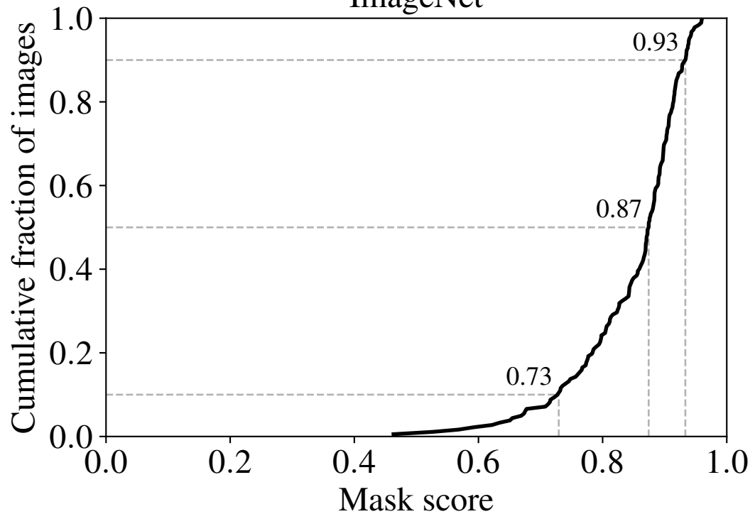
ImageNet
