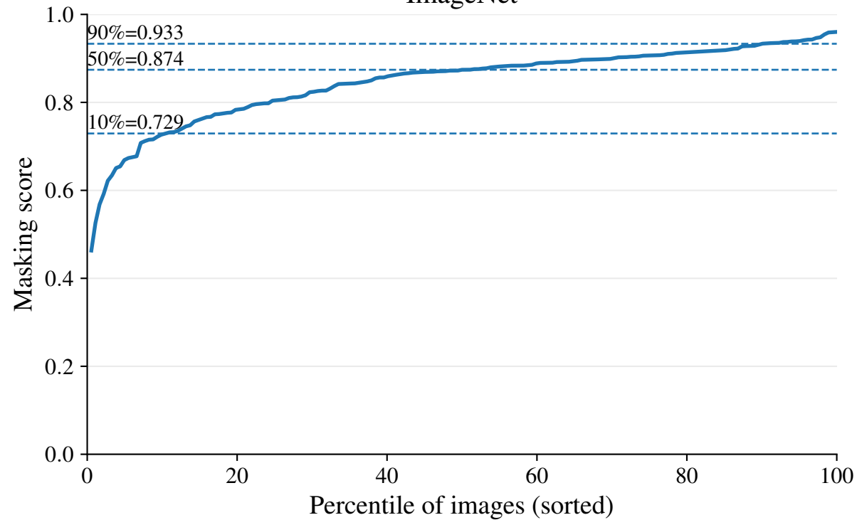
ImageNet
