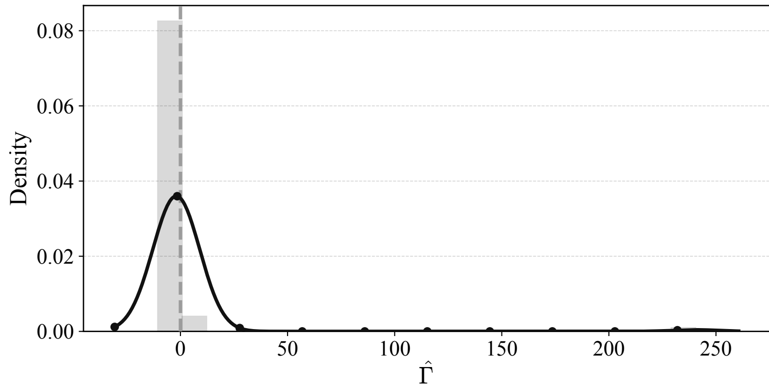
ImageNet
