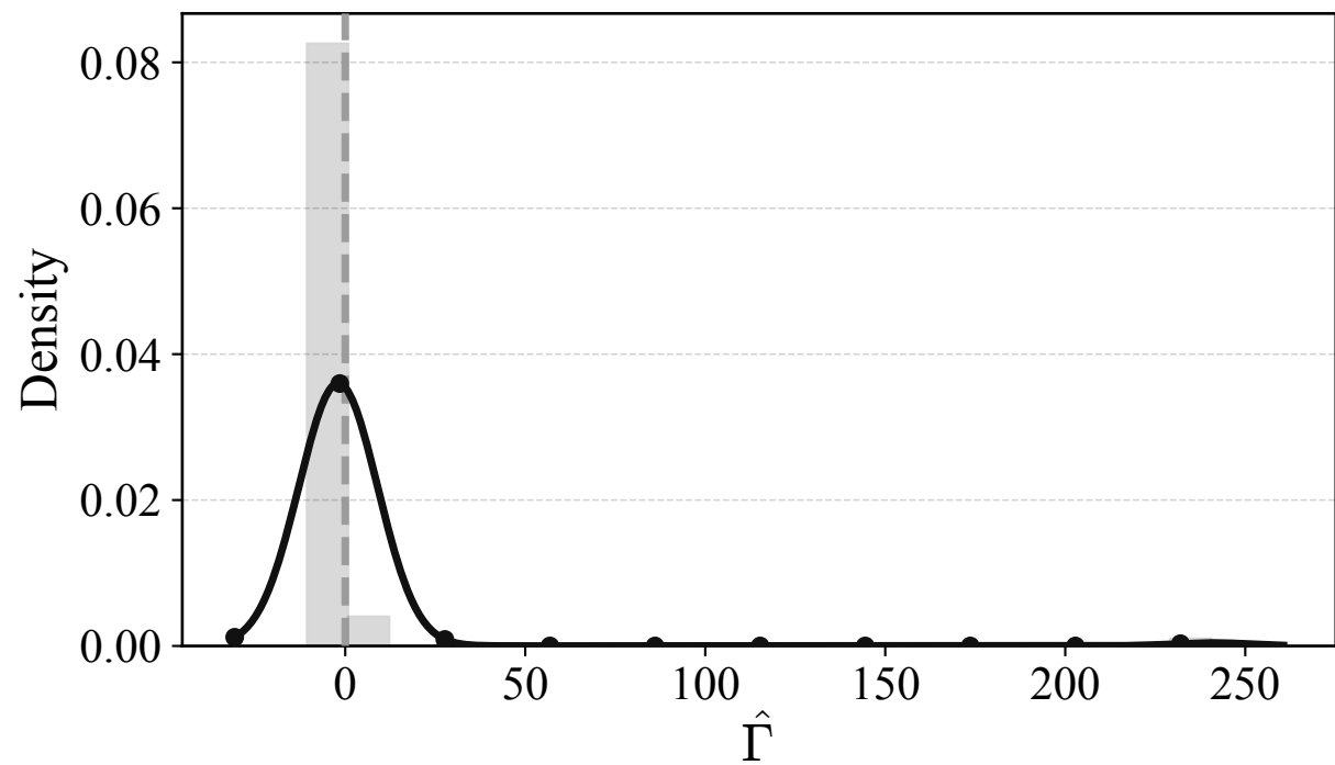
ImageNet
