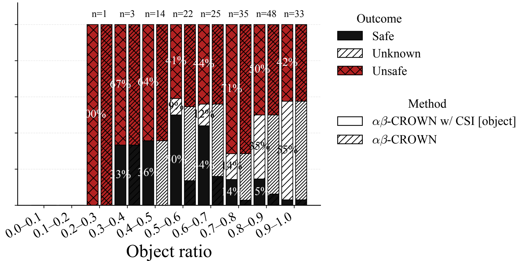
ImageNet
