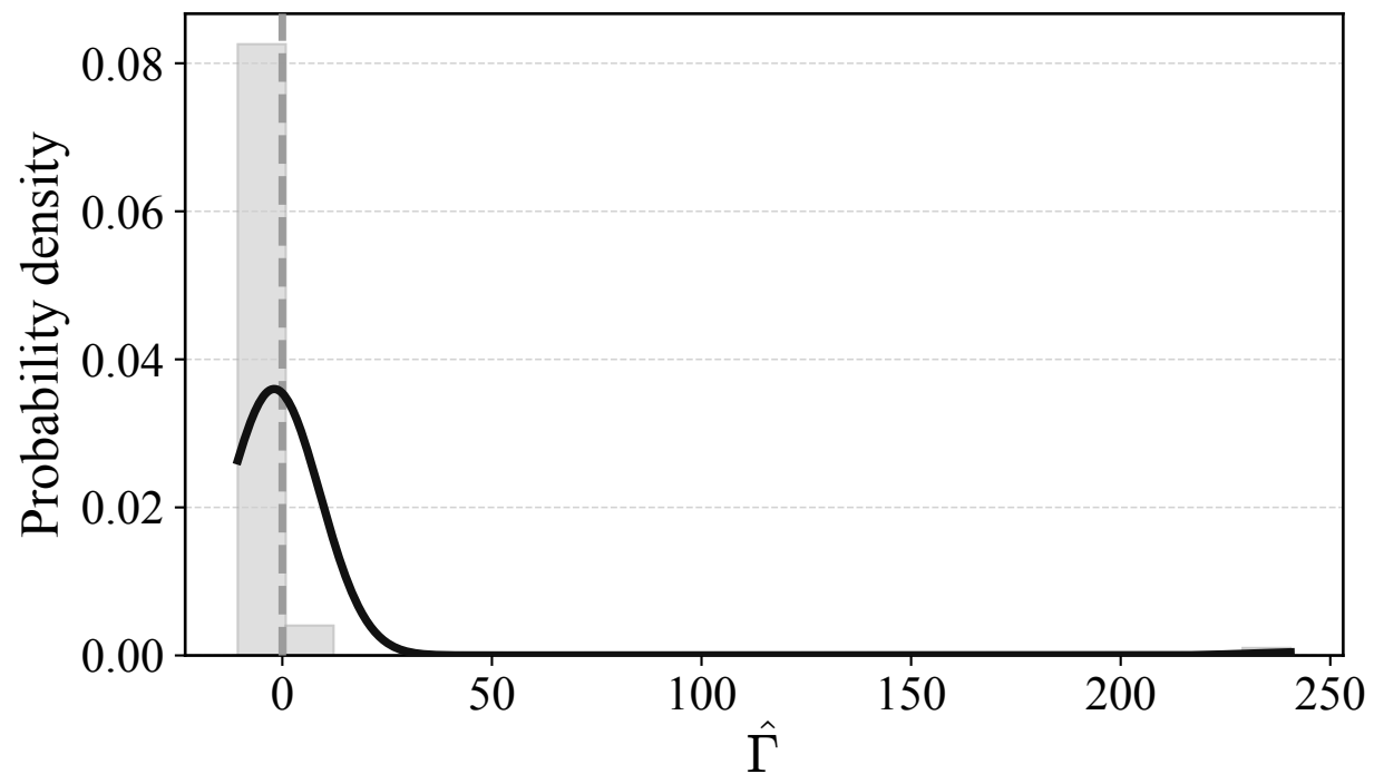
ImageNet
