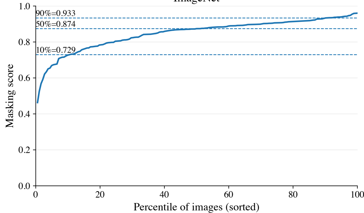
ImageNet
