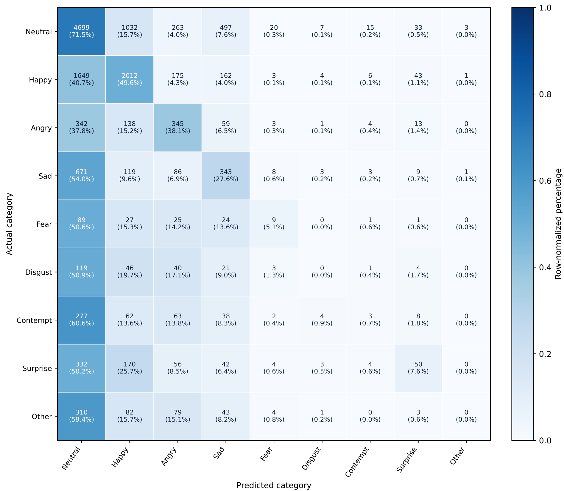
MH KLD · Test2
