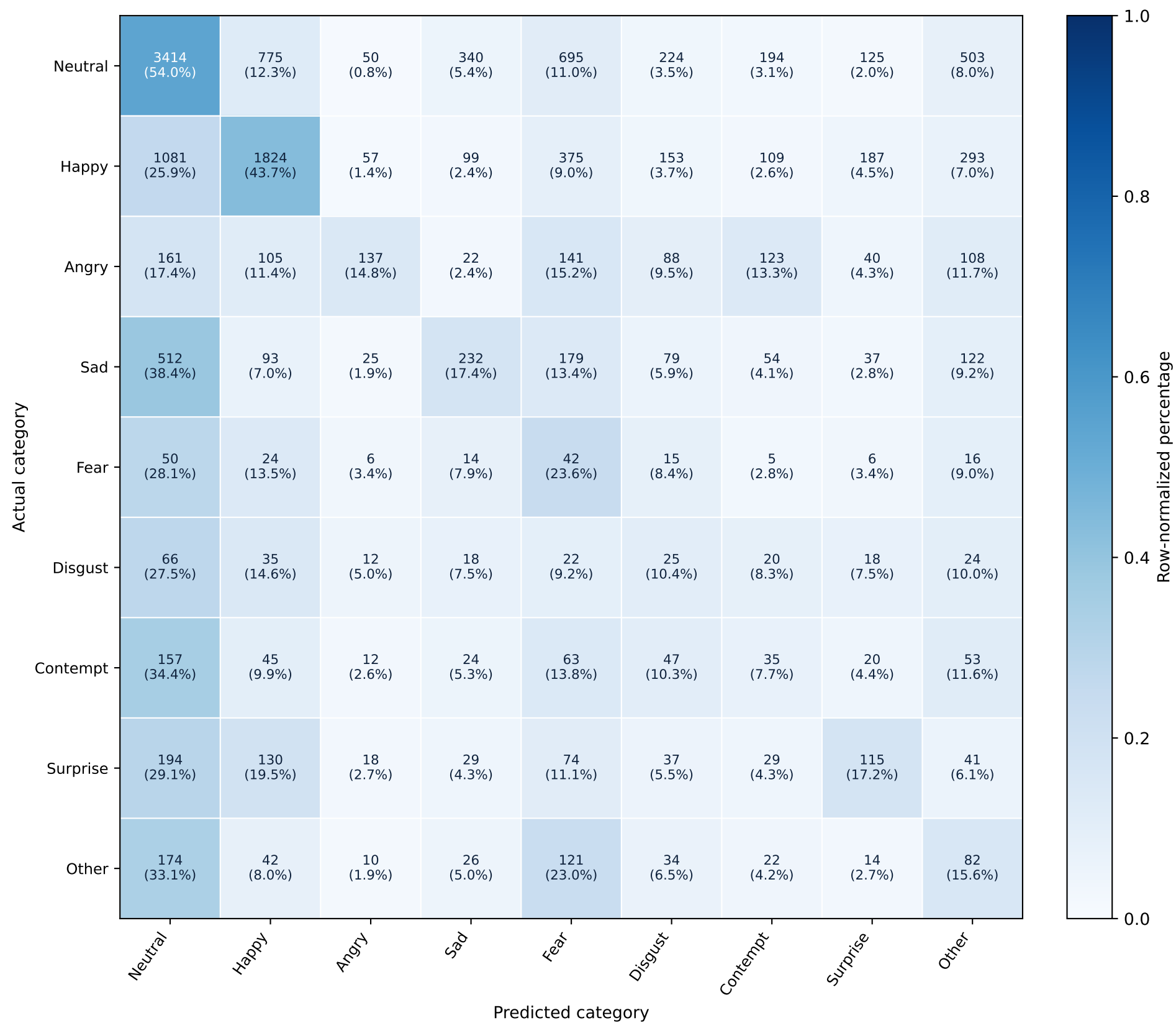
ML KLD · Test2
