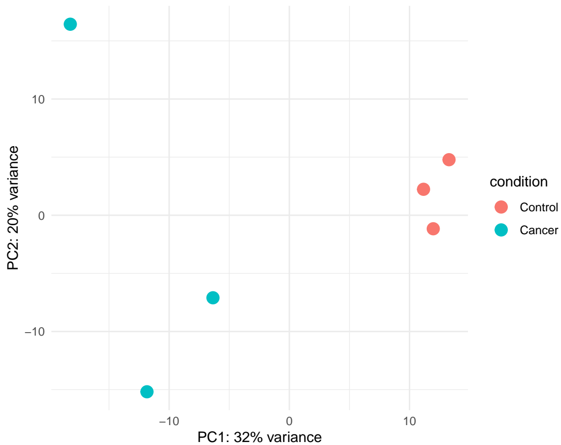
PCA plot
