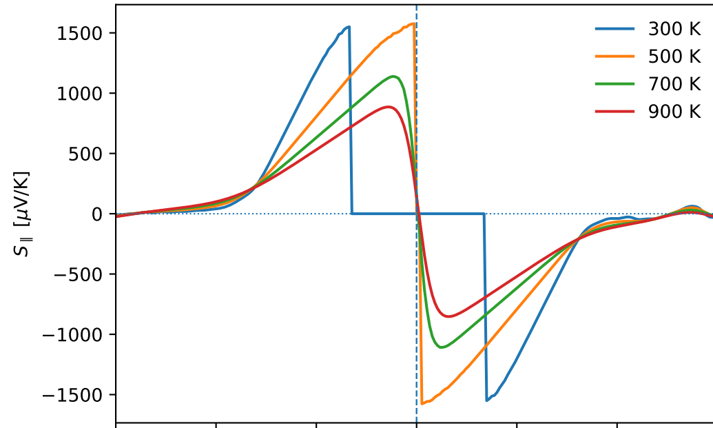
Koefisien Seebeck
