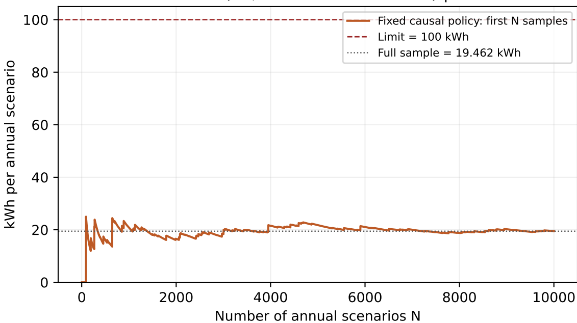
Validation (10,000 annual scenarios) | EENS
