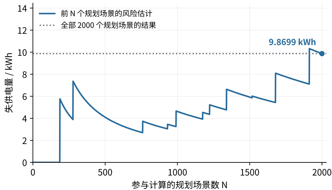
EENS | 约束上限 100 kWh
