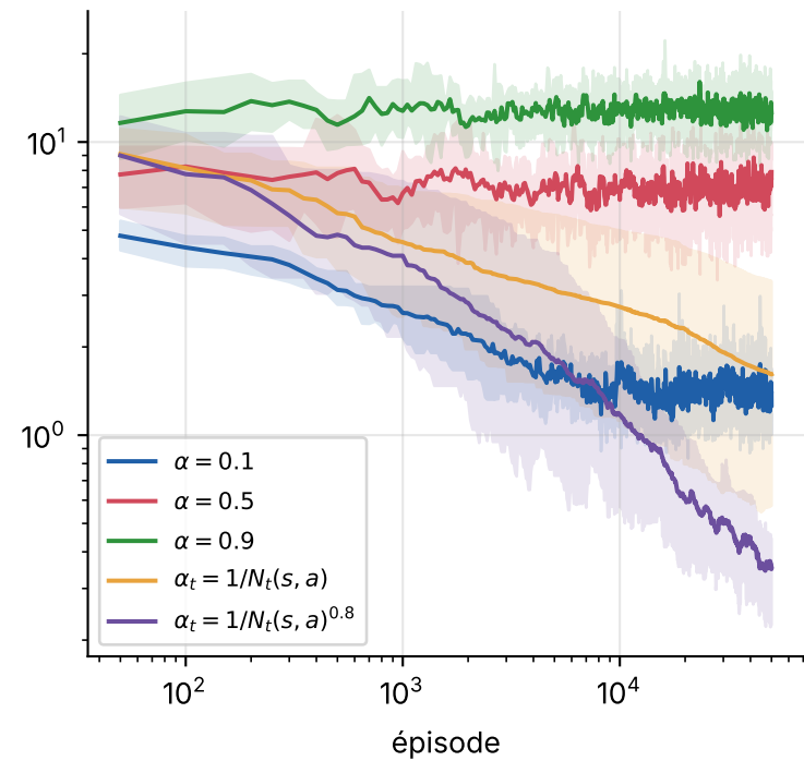
Q-Learning : \|Q_t - Q^*\|_\infty
