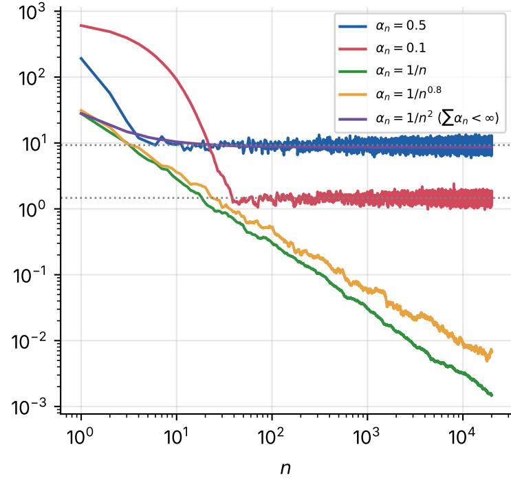
Robbins-Monro scalaire : \mathbb{E}[(x_n - m)^2] (200 répétitions)
