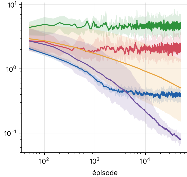
Q-Learning : moyenne de |Q_t - Q^*|
