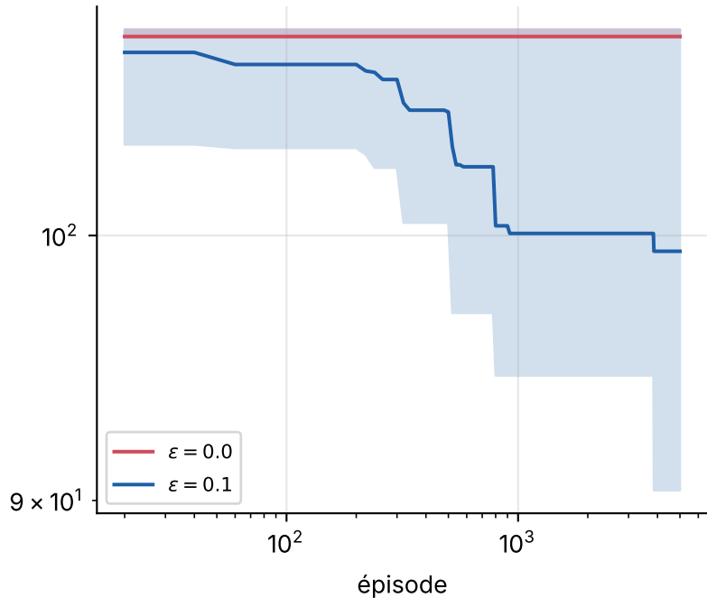
\|Q_t - Q^*\|_\infty , initialisation pessimiste
