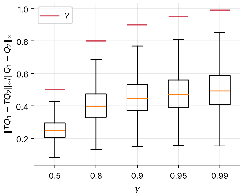
Contraction : 20 000 couples aléatoires par \gamma
