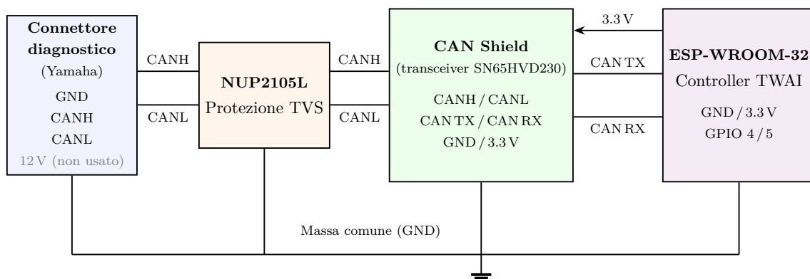
Figura 5.16: Schema elettrico di EggLog CAN Sniffer.
