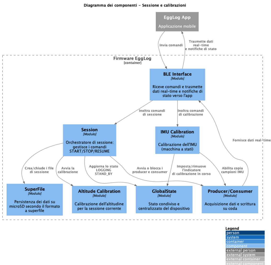
Figura 5.11: Diagramma dei componenti del firmware EggLog: sessione e calibrazioni
