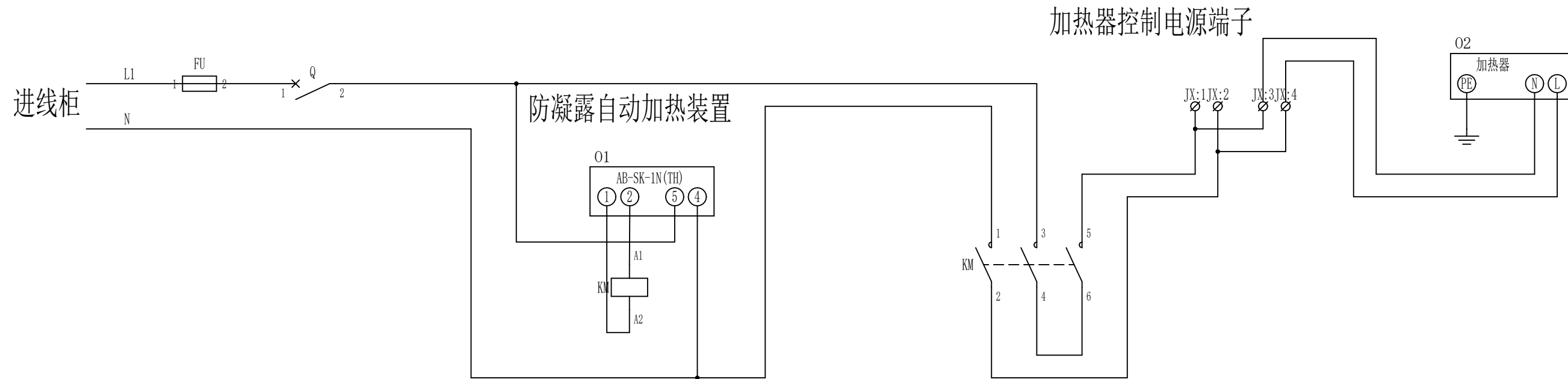
适用于进线柜
