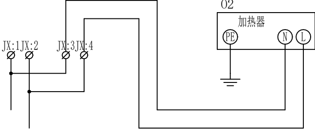
加热器控制电源端子
