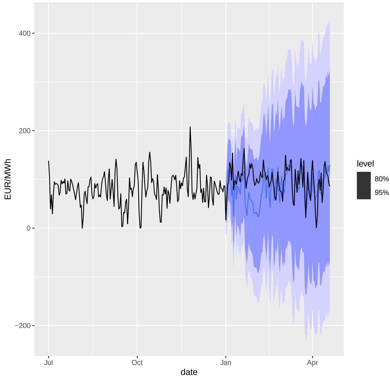
Dynamic regression (wind) forecast vs actual
