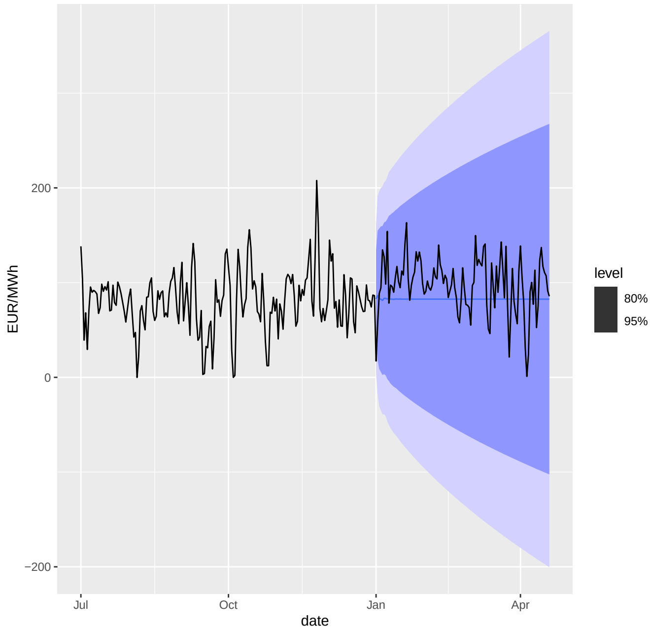
Auto-ARIMA forecast vs actual
