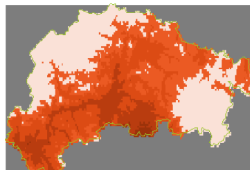
Mean temp. 2071-2100
