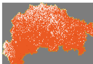
Precipitation 2071-2100
