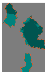
Sommerniederschlag 2071-2100
