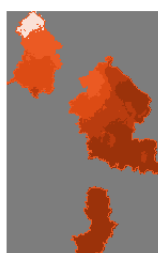
Mitteltemp. 2071-2100
