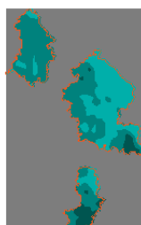
Sommerniederschlag Basiswert
