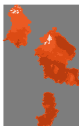
Niederschlag Basiswert
