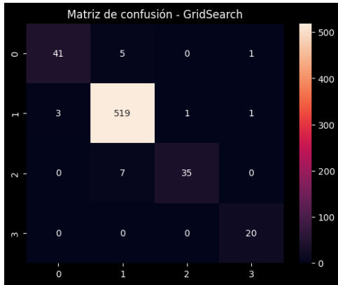
(b) RF con GridSearch
