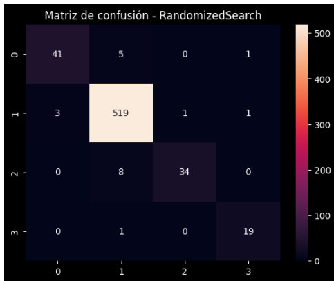
(c) RF con RandomizedSearch
